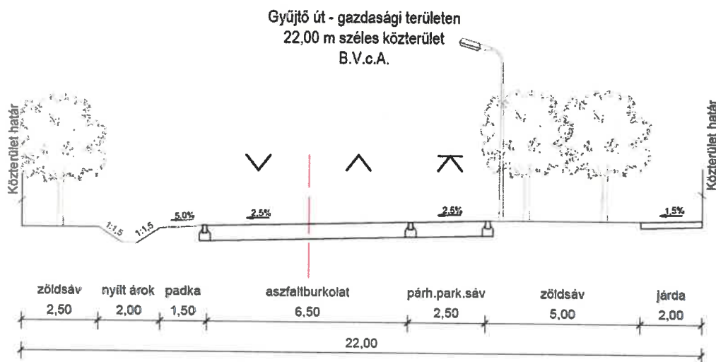
Mintakeresztmetszelvény – Gyűjtőút (belterület, 22 m széles)
