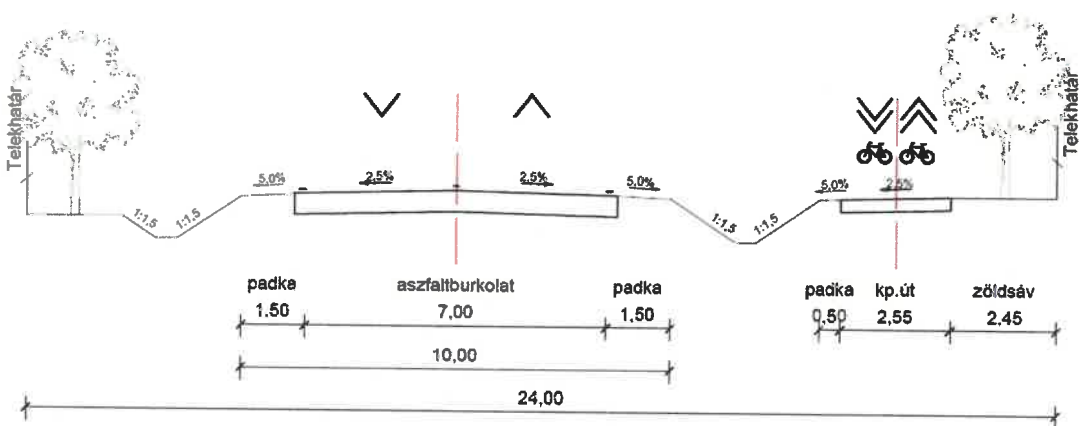
Mintakeresztszelvény – országos mellékút, külterületi szakasz kerékpárúttal (24 m széles)
