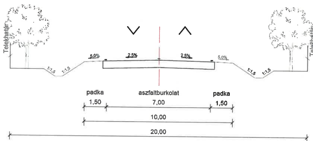
Mintakeresztszelvény – országos mellékút, külterületi szakasz (20 m széles)
