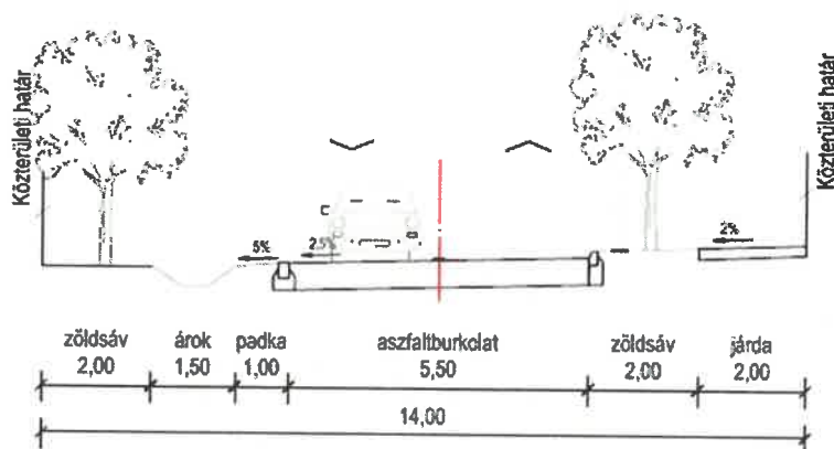
Mintakeresztmetszvény – Belterületi kiszolgáló út (14 m széles)
