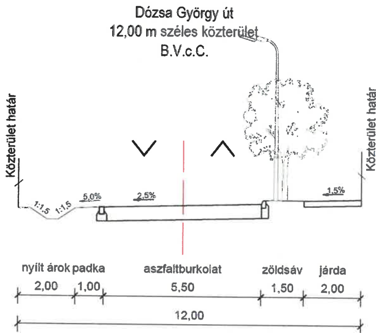
Mintakeresztmetszelvény – Dózsa György út (belterület, 12 m széles)
